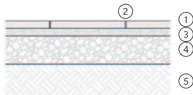
Lapok fektetése kavicságyra (csak gyalogos forgalmú felületek)
